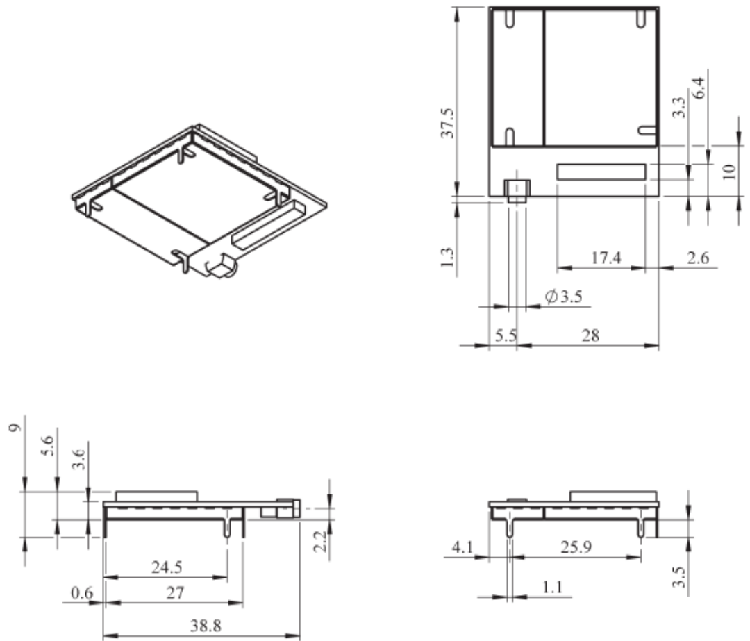
Fig. 2.2.1.1 TM2 Dimensional layout
