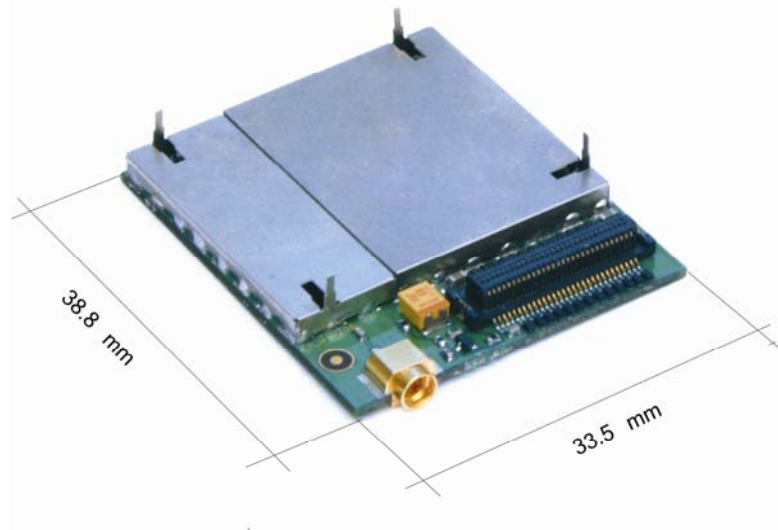
3.1 Fig. TM2 module
